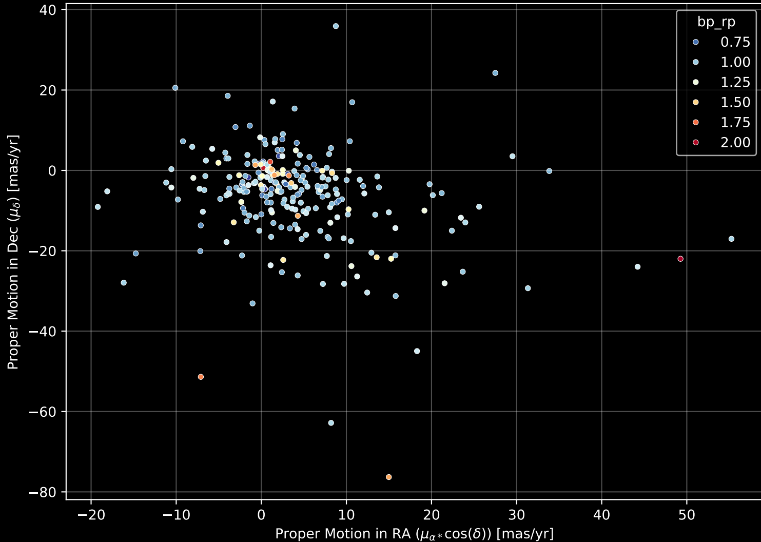
GALAH DR4 Field: [1303] Proper Motion Diagram (n= 255)
