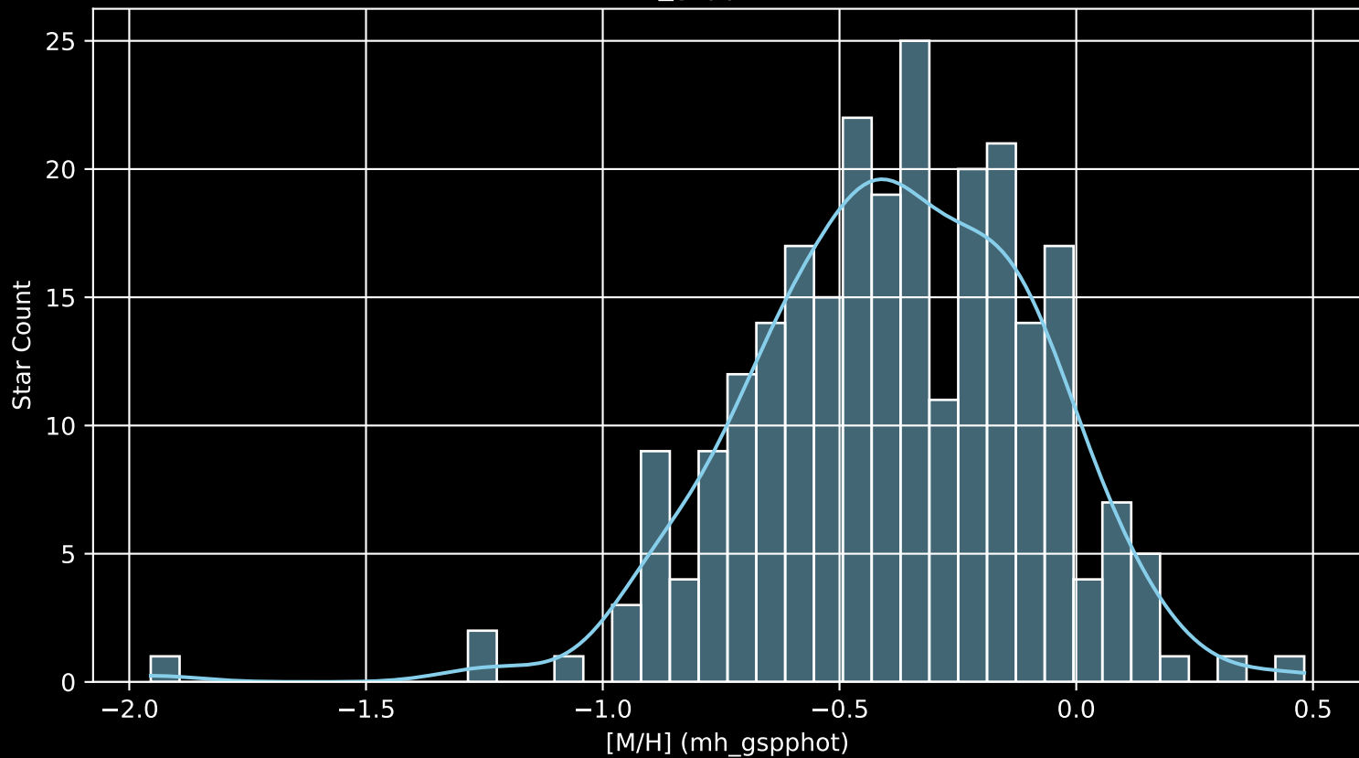
GALAH DR4 Field: [1303] [M/H] (mh_gspphot) (n= 255)
