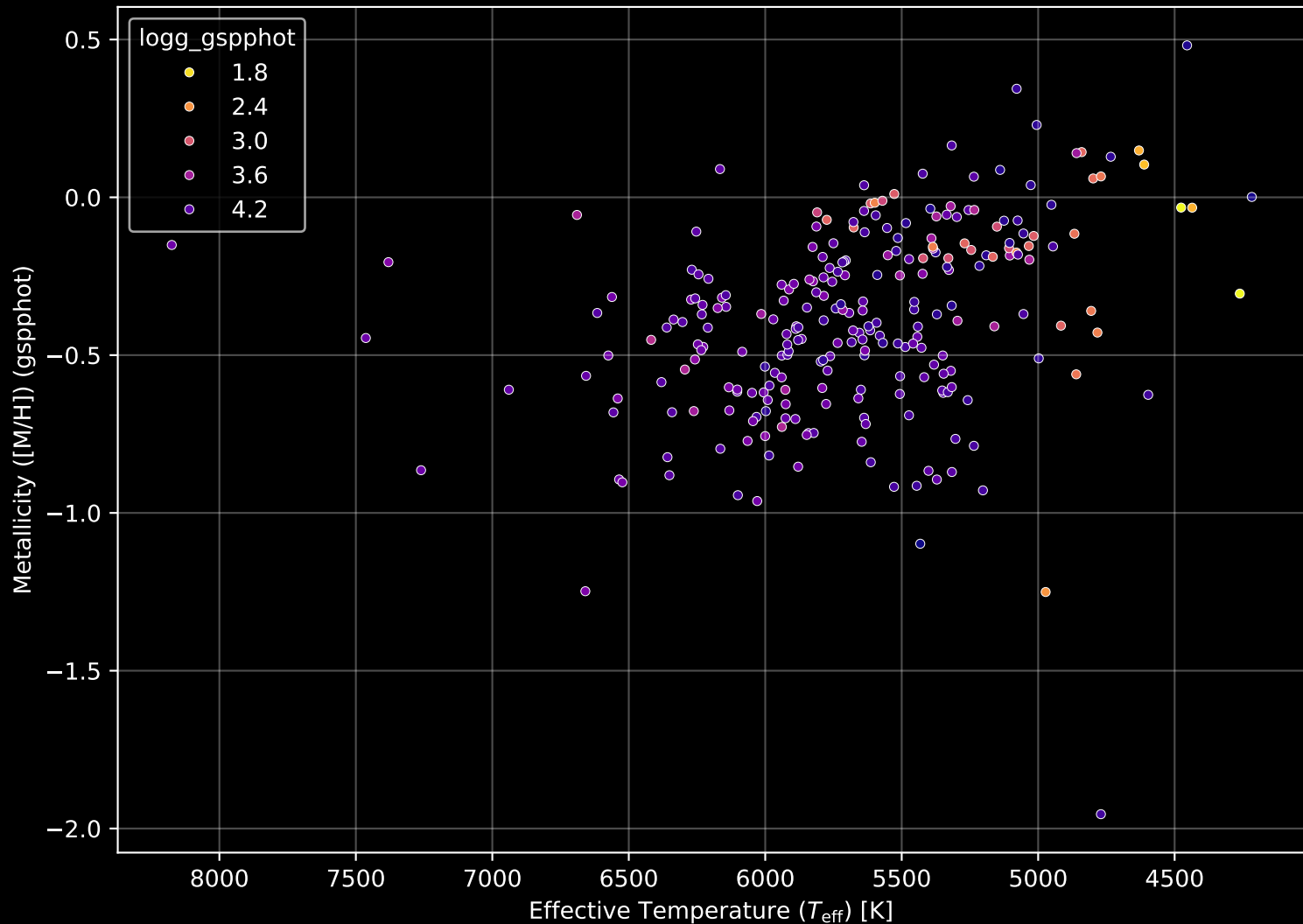
GALAH DR4 Field: [1303] Stellar Population Parameters (n= 255)
