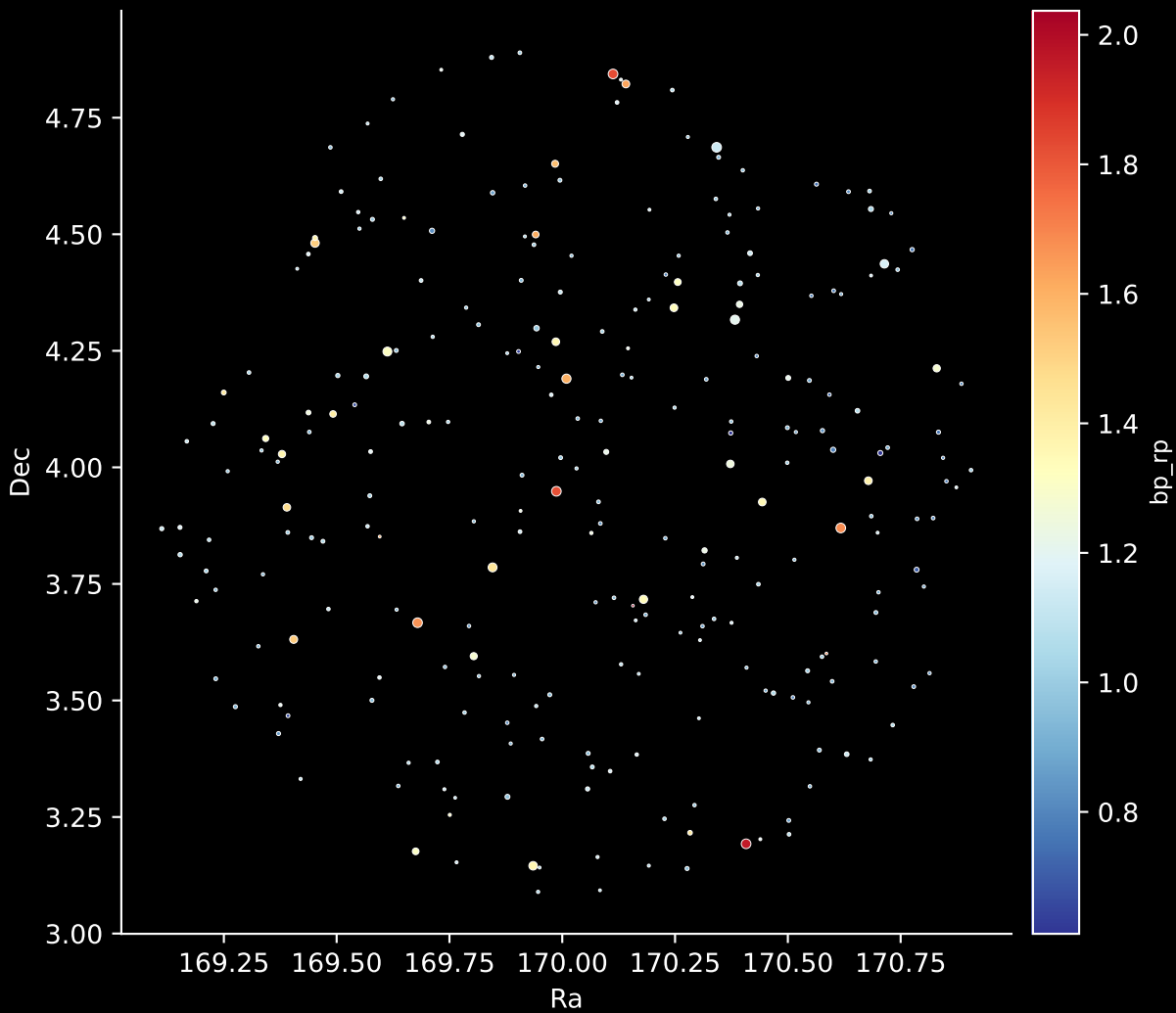
GALAH DR4 Field: [1303] Stars: 255
