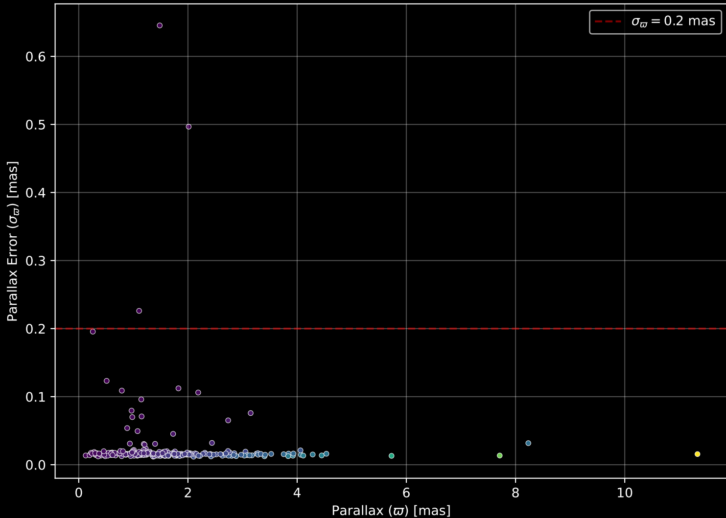
GALAH DR4 Field: [1303] Parallax Quality (n= 255)
